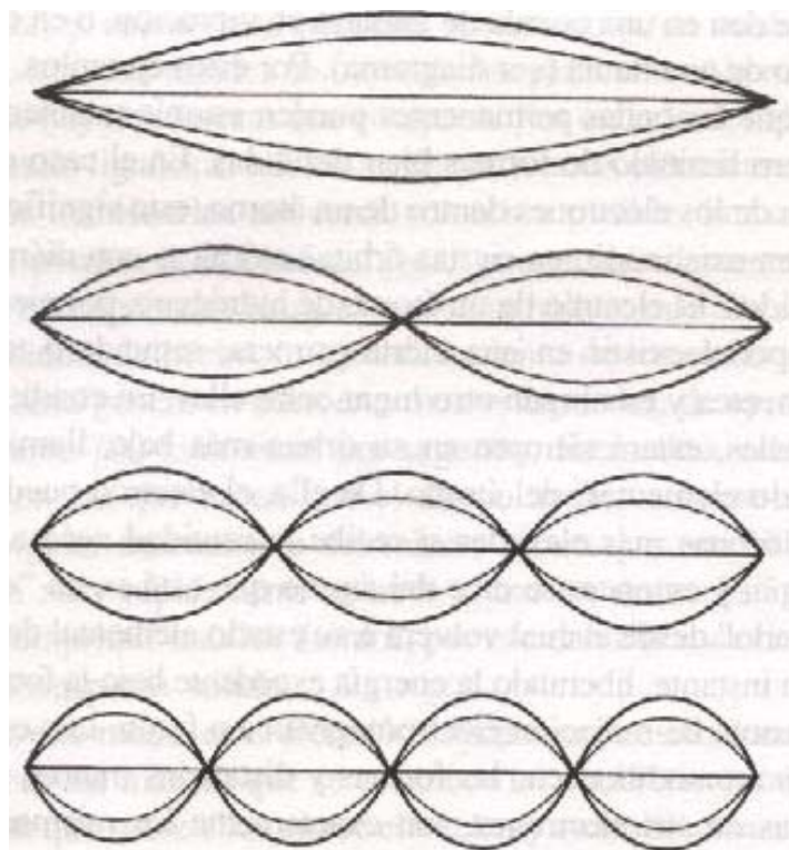
Patrones de onda permanente en la vibración de una cuerda
