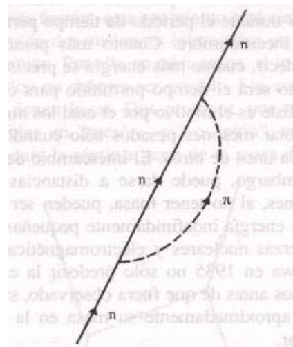
Un neutrón (n) que emite y reabsorbe un pión.
