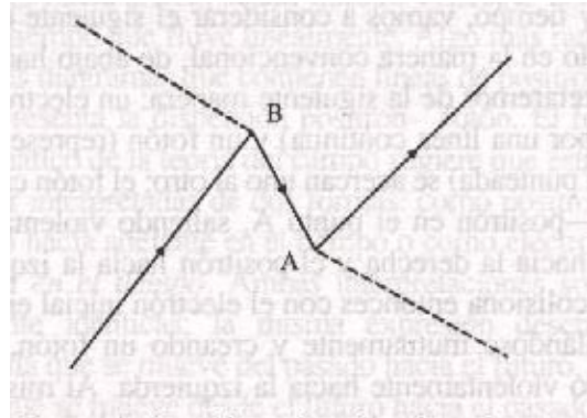
Proceso de dispersión en el que intervienen fotones, electrones y un positrón.
