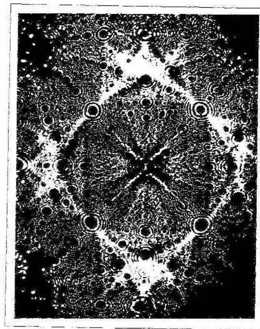
Con el microscopio electrónico se comprueba la distribución regular de los átomos en un cristal de platino. Pero, ¿observamos realmente los átomos o simples manchas en una placa fotográfica?
