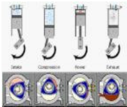
Motor Wankel
