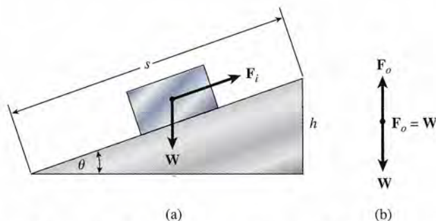
Figura 12.12 El plano inclinado. La fuerza de entrada representa el esfuerzo requerido para empujar el bloque hacia arriba por el plano; la fuerza de salida es igual al peso del bloque.
