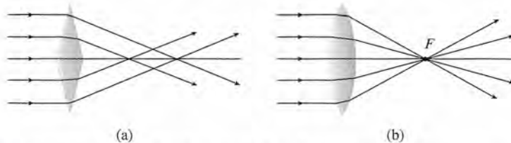
Figura 36.2 (a) Dos prismas colocados base contra base hacen convergir los rayos pero no los conducen hacia un foco común. (b) Una lente convergente puede construirse curvando uniformemente las superficies.
