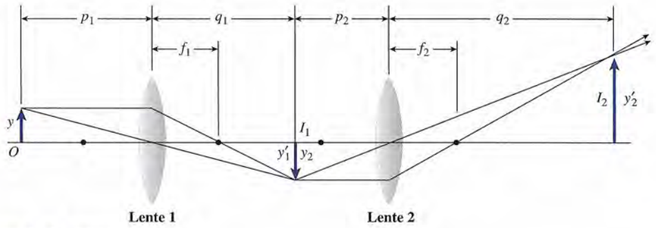
Figura 36.14 El microscopio.
