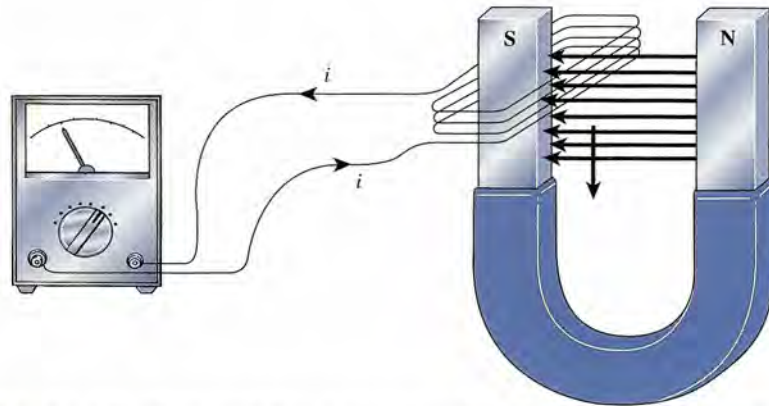
Figura 31.2 La fem inducida en una bobina es proporcional al número de espiras de alambre que cruzan a través del campo.
