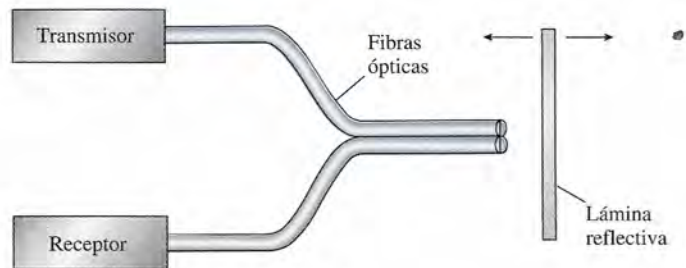
Figura 35.14 Sensor de desplazamiento de fibra óptica.
