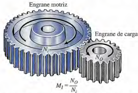
Figura 12.10 Engranes cilíndricos. La ventaja mecánica ideal es la razón del número de dientes del engrane de salida al número de dientes del engrane de entrada.
