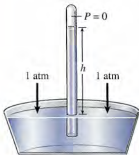
Figura 15.8 Barómetro.
