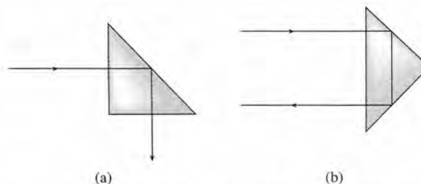
Figura 35.10 Los prismas de ángulo recto hacen uso del principio de reflexión interna total para desviar la trayectoria de la luz.
