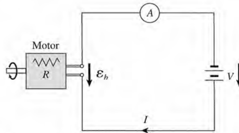
Figura 31.12 Fuerza contraelectromotriz en un motor de cd.
