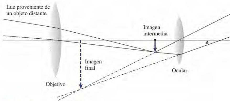
Figura 36.16 Telescopio de refracción.
