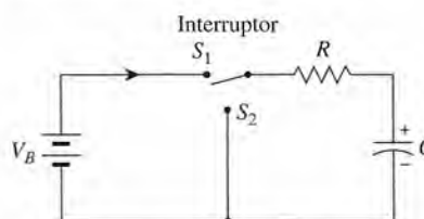
Figura 32.1 Diagrama de un circuito que muestra un método para cargar y descargar un condensador.
