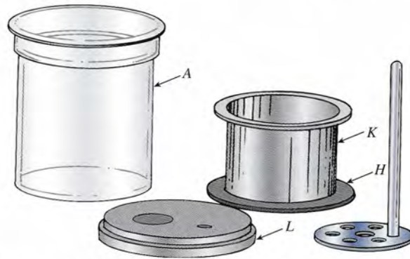
Figura 17.4 El calorímetro de laboratorio. (Central Scientific Co.)
