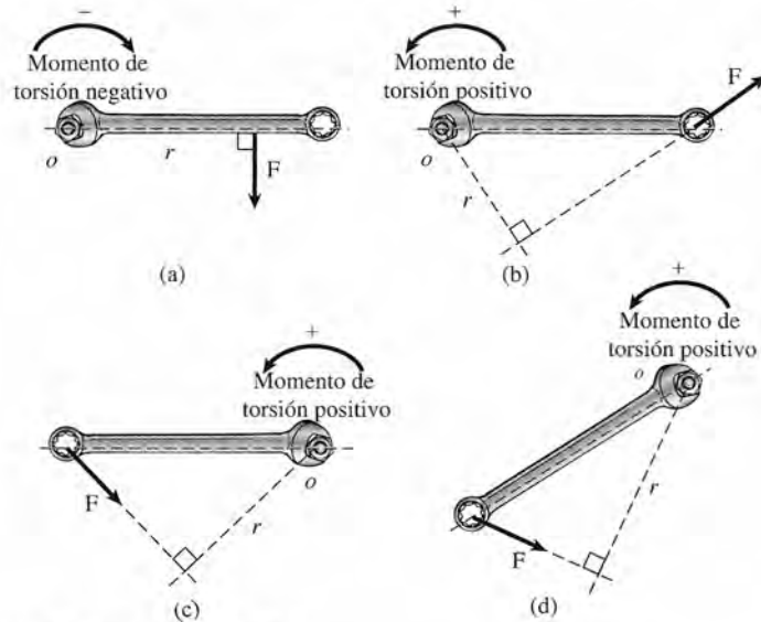
Figura 5.3 Ejemplos de brazos de palanca r .
