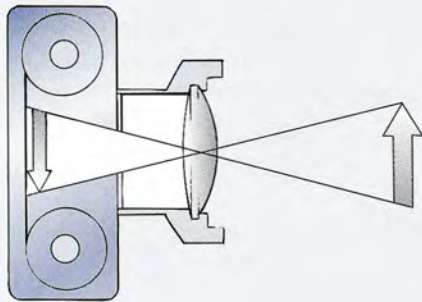
Figura 36.19 La cámara.
