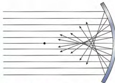
Figura 34.16 Aberración esférica.
