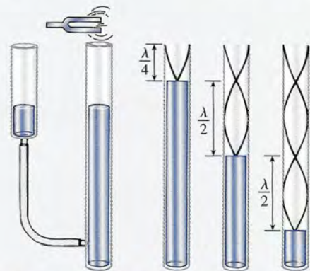
Figura 22.16 Aparato de laboratorio para calcular la velocidad del sonido mediante el método de resonancia.
