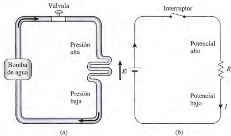
Figura 27.4 La analogía mecánica de una bomba de agua resulta útil para explicar la función de una fuente de fem en un circuito eléctrico.
