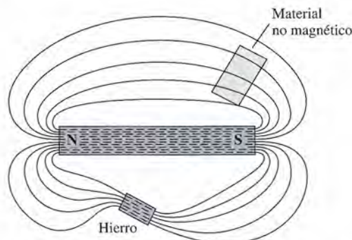
Figura 29.11 Un material permeable se magnetiza por inducción, lo que da por resultado una mayor densidad de flujo en esa región.
