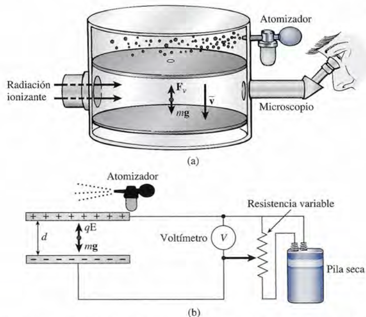
Figura 25.10 Experimento de Millikan de la gota de aceite: (a) La masa m de la gota se determina a partir de su velocidad de caída, en contra de la fuerza viscosa de la resistencia del aire. (b) La magnitud de la carga se puede calcular partiendo de las condiciones de equilibrio que mantienen suspendida la carga entre dos placas con carga opuesta (véase la figura 25.10).
