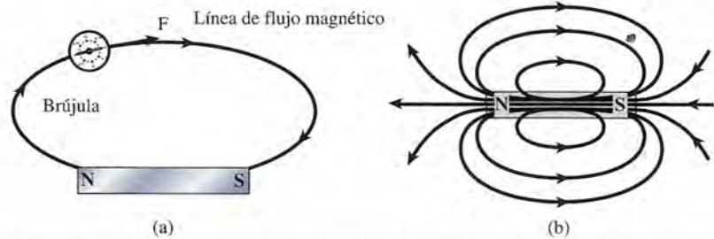
Figura 29.4 (a) Las líneas de flujo magnético están en la dirección de la fuerza que se ejerce sobre un polo norte independiente. (b) Las líneas de flujo cercanas a una barra imantada.
