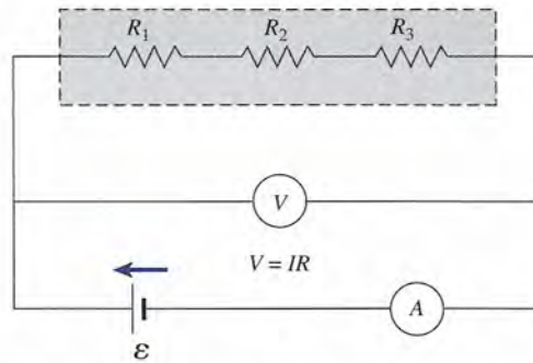
Figura 28.3 Método del voltímetro-amperímetro para medir la resistencia efectiva de varios resistores conectados en serie.
