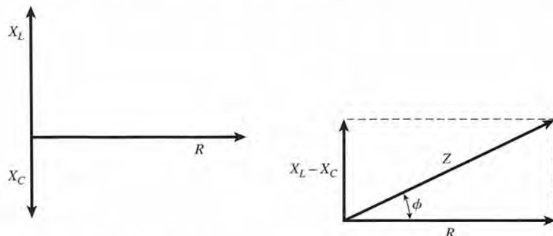
Figura 32.12 Diagrama de la impedancia.
