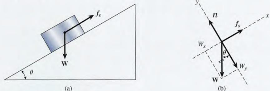
Figura 4.17 El ángulo de reposo o limitante.
