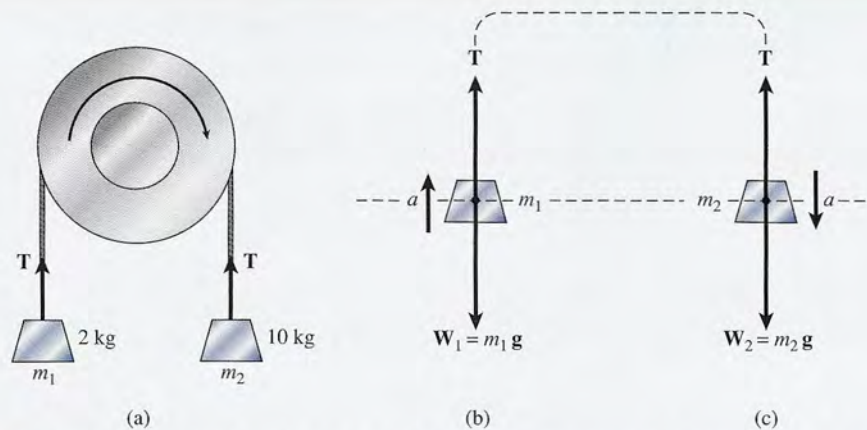
Figura 7.8 Dos masas cuelgan de una polea fija. Se muestran los diagramas de cuerpo libre; la dirección positiva de la aceleración se elige hacia arriba a la izquierda, y hacia abajo a la derecha.
