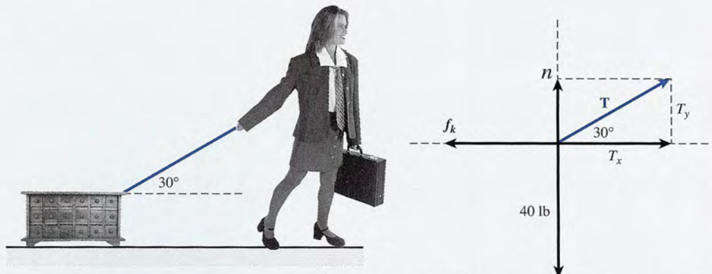
Figura 4.15 La fuerza \mathbf{T} en un ángulo sobre la horizontal reduce la fuerza normal necesaria para el equilibrio, lo que ocasiona que la fuerza de fricción sea menor. (Fotografías de Hemera Inc.)
