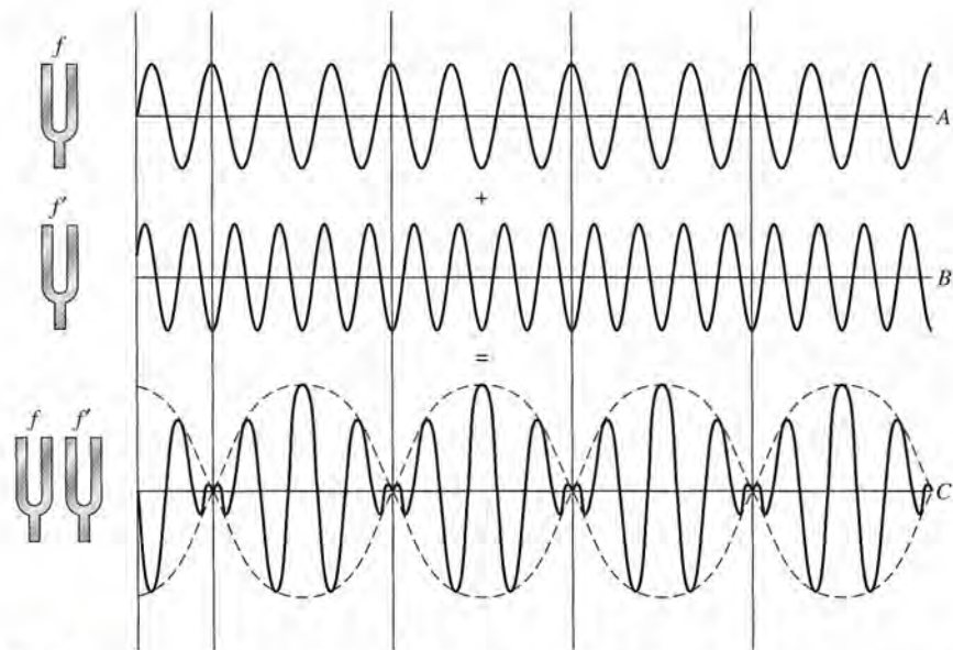
Figura 22.10 Diagrama que muestra el origen de las pulsaciones. La onda C es una superposición de ondas A y B.
