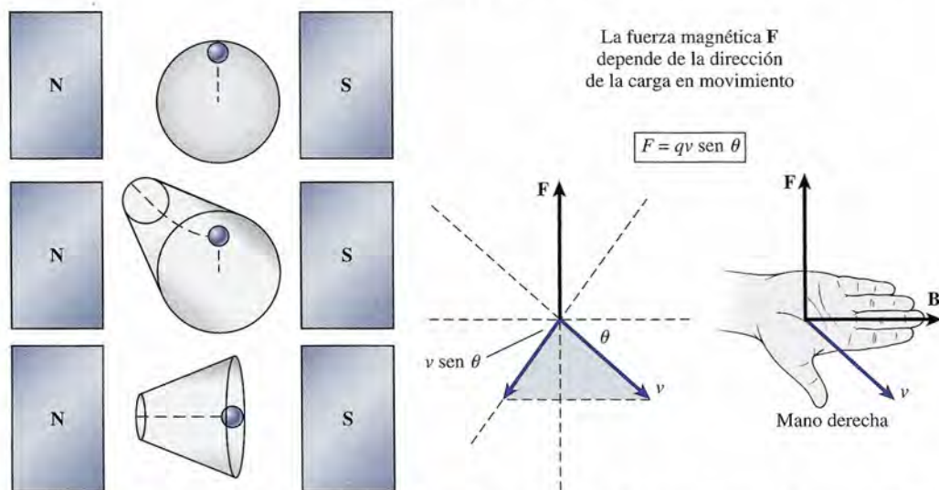
Figura 29.15 La magnitud de la fuerza magnética adquiere su valor máximo cuando la trayectoria es perpendicular al campo y su valor mínimo cuando es paralela al mismo.
