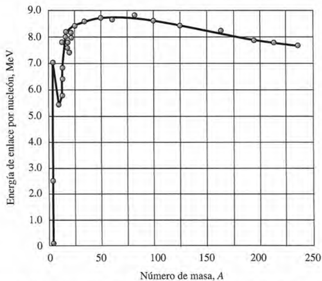
Figura 39.4 La energía de enlace media por nucleón para los núcleos más estables en relación con el número de masa.
