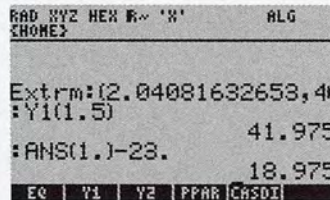
Figura 11. La altura después de 1.5 segundos.
