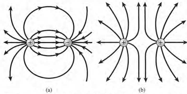
Figura 24.9 (a) Diagrama de las líneas del campo eléctrico en la región que rodea dos cargas opuestas. (b) Las líneas del campo entre dos cargas positivas.
