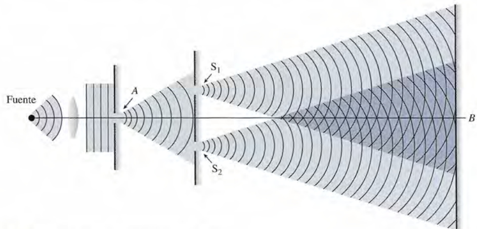
Figura 37.2 Ilustración del experimento de Young.
