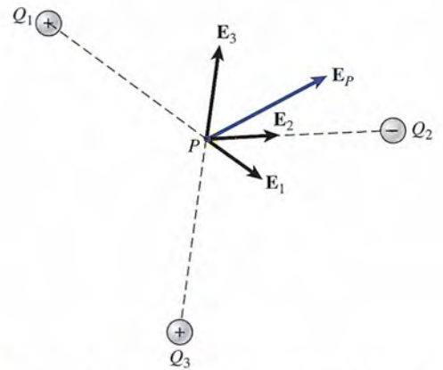
Figura 24.6 El campo en la proximidad de varias cargas es igual a la suma vectorial de los campos debido a las cargas individuales.
