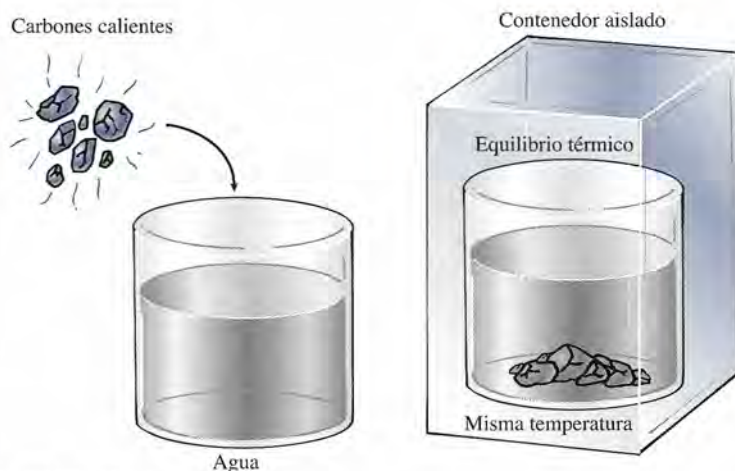
Figura 16.2 Equilibrio térmico.
