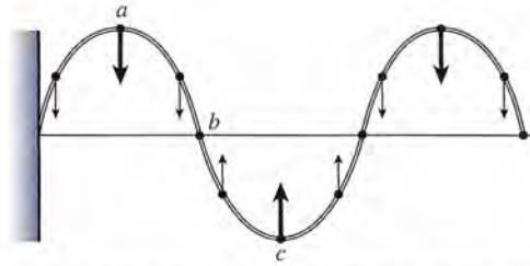
Figura 21.8 Fuerzas de restitución que actúan sobre las partículas de una cuerda vibrante.
