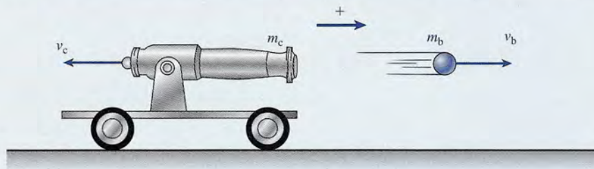
Figura 9.4 Cálculo de la velocidad de retroceso de un cañón.
