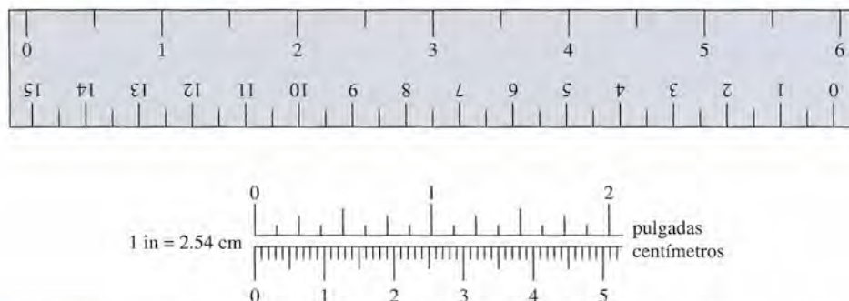
Figura 3.1 Comparación de la pulgada con el centímetro como medidas de longitud.
