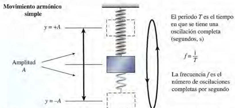
Figura 14.3 El movimiento armónico simple (MAS) es un movimiento periódico con amplitud, frecuencia y periodo constantes.
