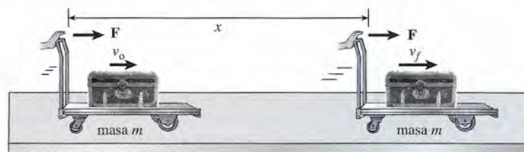
Figura 8.4 El trabajo realizado por la fuerza resultante \mathbf{F} produce un cambio en la energía cinética de la masa total m . (Fotografías de Hemera.)
