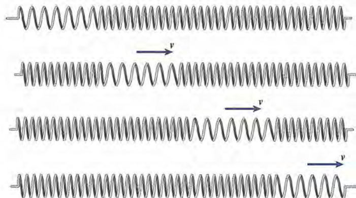
Figura 21.3 Movimiento longitudinal de un pulso de rarefacción en un resorte en espiral.
