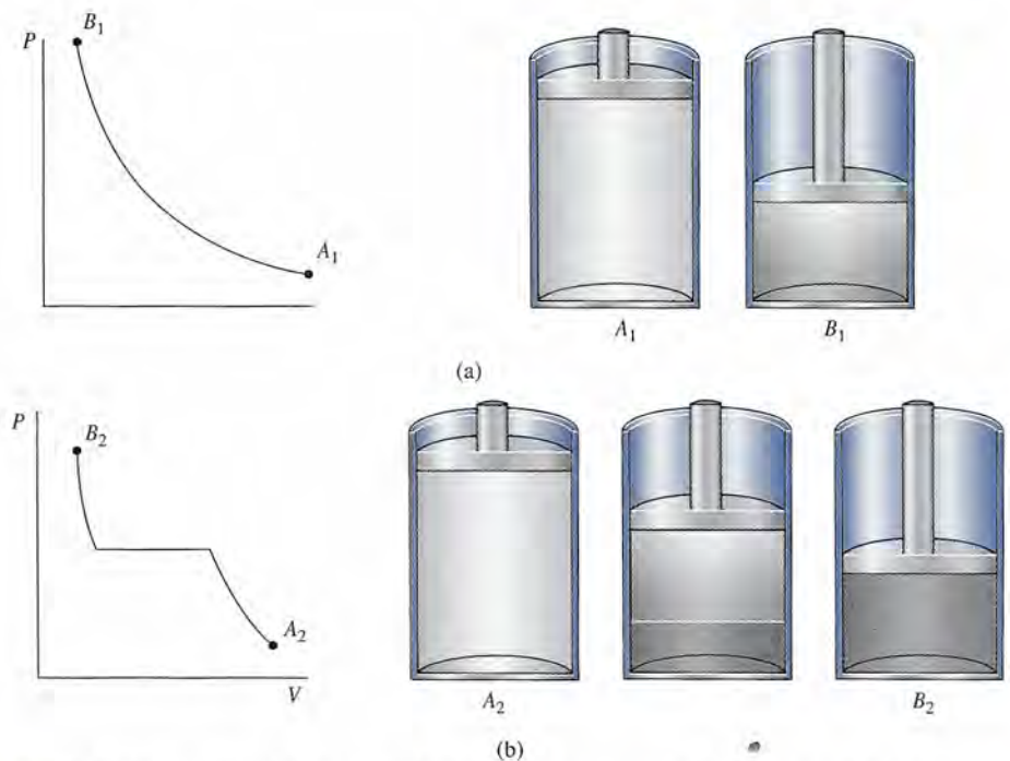
Figura 19.4 (a) Compresión de un gas ideal a cualquier temperatura o de un gas real a alta temperatura. (b) Licuefacción de un gas real cuando se comprime a bajas temperaturas.
