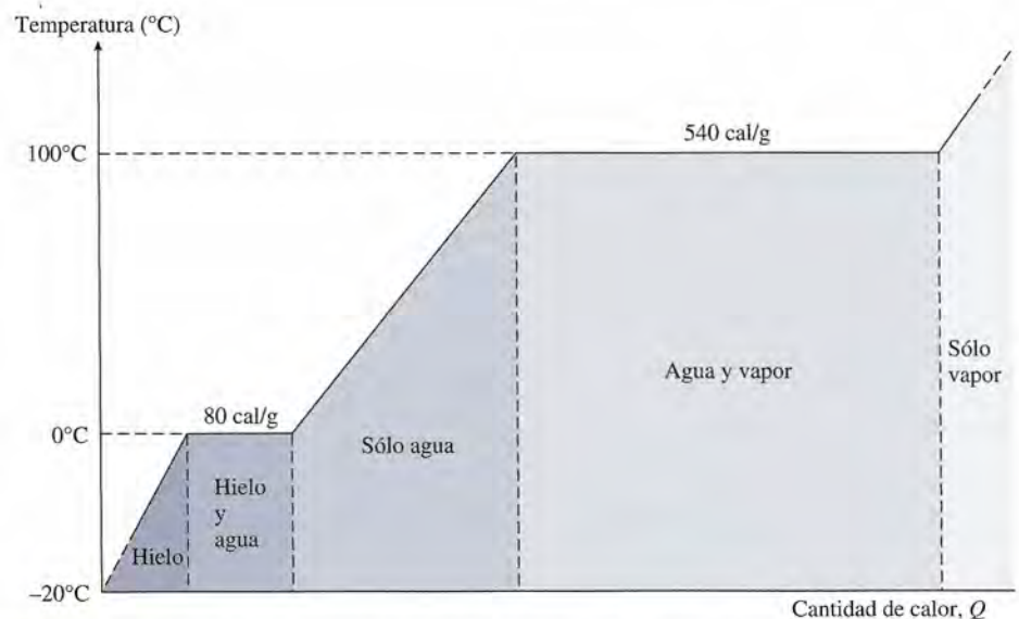
Figura 17.7 Variación de temperatura debida a un cambio de la energía térmica del agua.
