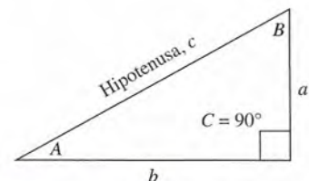
Figura 2.12 En un triángulo rectángulo uno de los ángulos internos debe ser recto.
