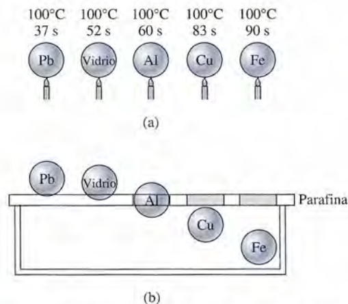
Figura 17.3 Comparación entre las capacidades caloríficas de cinco esferas de materiales diferentes.
