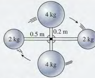
Figura 11.6 Cálculo del momento de inercia.
