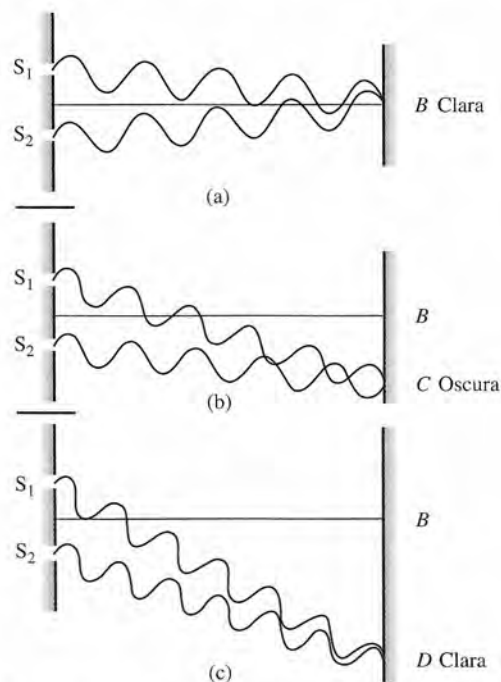
Figura 37.4 Origen de las bandas claras y oscuras en un patrón de interferencia.
