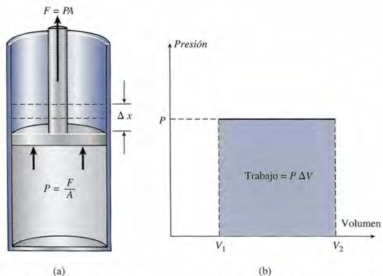
Figura 20.4 (a) Cálculo del trabajo realizado por un gas que se dilata a presión constante. (b) El trabajo es igual al área debajo de la curva en un diagrama P-V.
