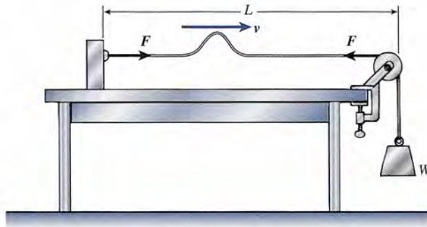
Figura 21.4 Cálculo de la rapidez de un pulso transversal en una cuerda.
