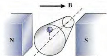
Figura 29.13 La fuerza magnética F sobre una carga en movimiento es perpendicular tanto a la densidad de flujo B como a la velocidad de carga v .
