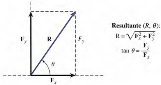
Figura 3.18 La resultante de dos vectores perpendiculares.
