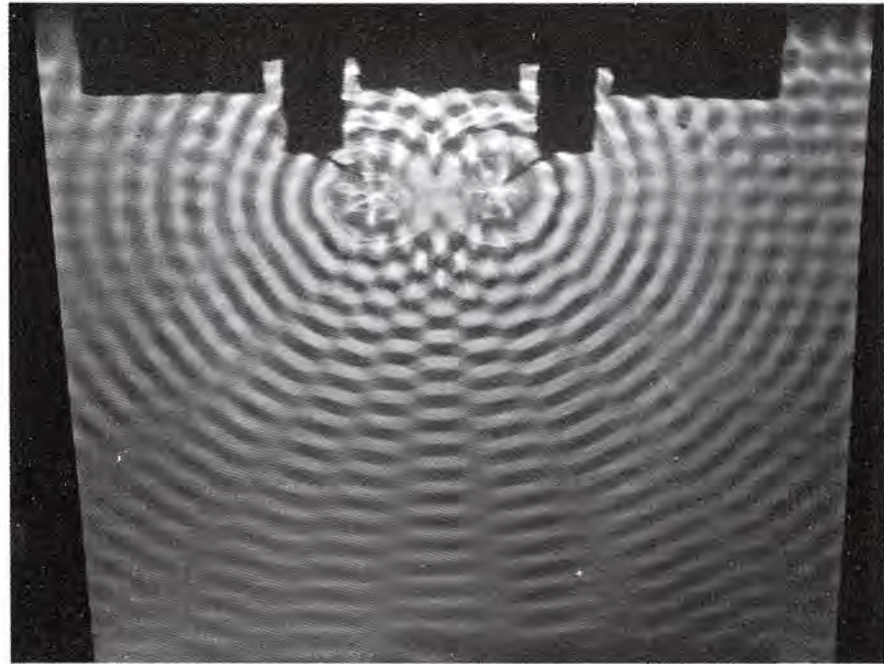
Figura 37.5 Patrón de interferencia de ondas en el agua formado por dos fuentes coherentes. (Tomado de PSCC Physics, D. C. Heath and Company, Lexington, Massachusetts, 1965).
