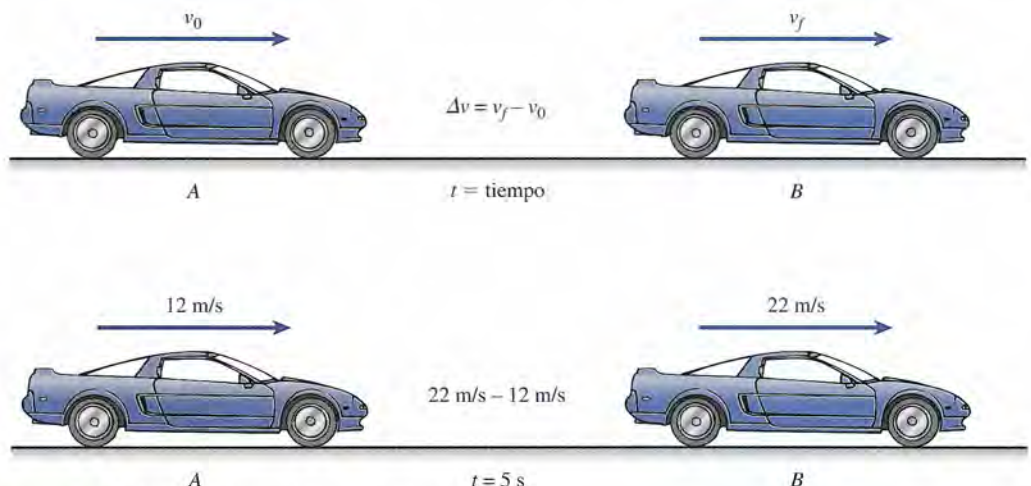
Figura 6.2 Movimiento uniformemente acelerado.
