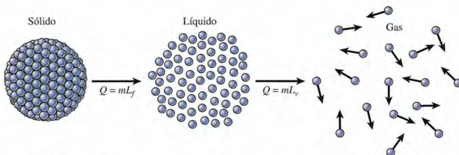
Figura 17.6 Un modelo simplificado muestra las separaciones moleculares relativas en las fases sólida, líquida y gaseosa. Durante un cambio de fase, la temperatura permanece constante.
