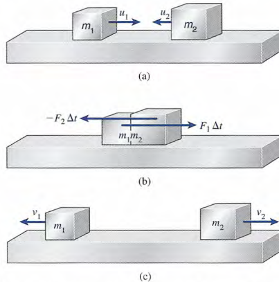
Figura 9.3 (a) Antes del impacto: m_1u_1 + m_2u_2 ; (b) durante el impacto F_1\Delta t = -F_2\Delta t ; (c) después del impacto m_1v_1 + m_2v_2 .
