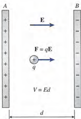
Figura 25.9 Potencial entre dos placas con cargas opuestas.
