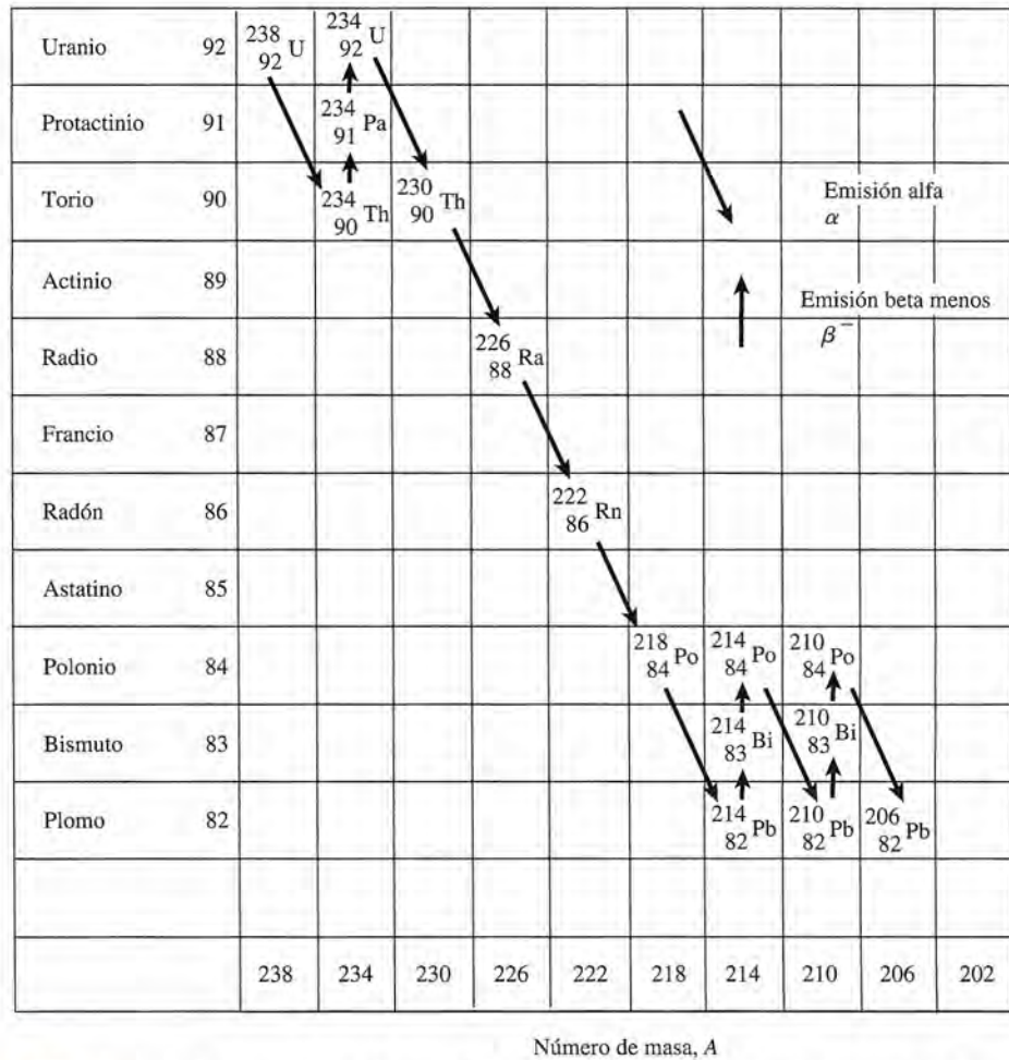
Figura 39.6 Serie de desintegración del uranio. Decaimientos del uranio, a través de una serie de emisiones alfa y beta negativa, de ^{238}\text{U} a ^{206}\text{Pb} .
