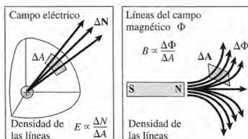
Figura 29.9 De igual forma en que el campo eléctrico es proporcional a la densidad de líneas del campo eléctrico, el campo magnético es proporcional a la densidad de las líneas de flujo del campo magnético.
