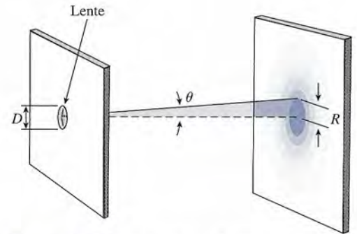
Figura 37.12 Límite de resolución.
