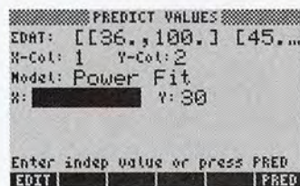
Figura 4. Antes de resolver x .
