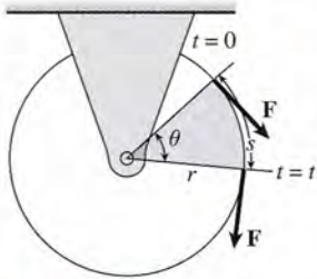
Figura 11.9 Trabajo y potencia en el movimiento de rotación.
