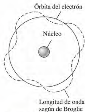
Figura 38.8 Órbita estable del electrón que muestra una circunferencia igual a cuatro longitudes de onda de de Broglie.
