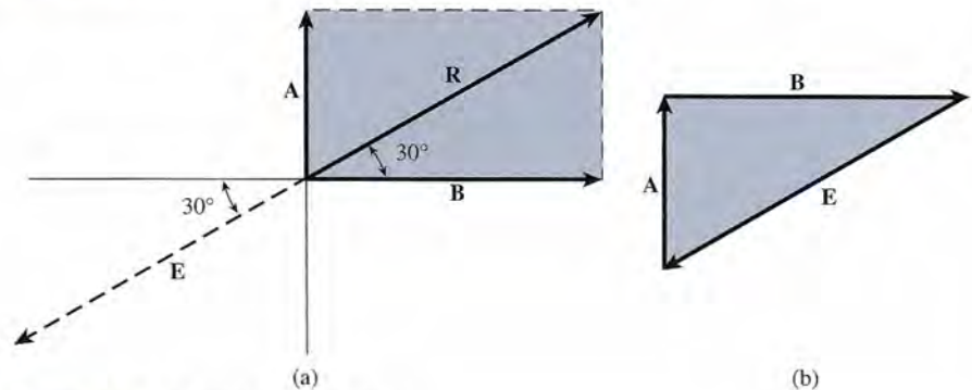
Figura 4.4 La fuerza equilibrante.
