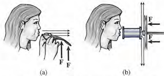
Figura 15.16 Demostraciones de la disminución de presión que resulta de un incremento en las rapidez del aire.
