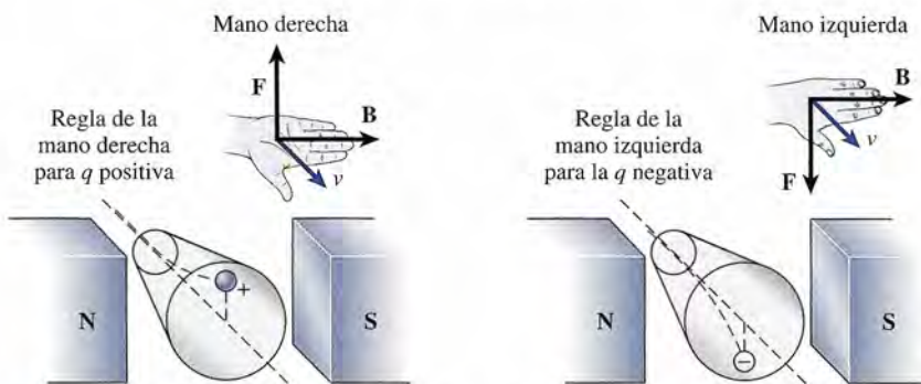
Figura 29.14 Uso de las reglas de la mano derecha y la mano izquierda para determinar la dirección de la fuerza magnética en una carga en movimiento. Los dedos apuntan en la dirección del campo B y el pulgar en la dirección de la carga en movimiento. La palma abierta está de cara a la dirección de la fuerza magnética F sobre una carga positiva. La mano derecha se usa para cargas positivas y la izquierda para cargas negativas.
