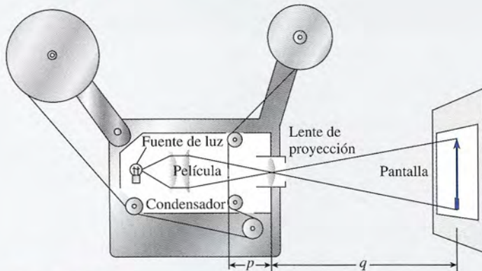
Figura 36.20 El proyector.
