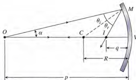
Figura 34.14 En un espejo convergente se forma una imagen puntual a partir de un objeto puntual.
