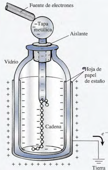
Figura 26.14 La botella de Leyden.
