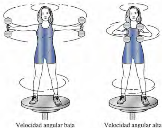
Figura 11.13 Experimento para demostrar la conservación de la cantidad de movimiento angular. La mujer controla su velocidad de rotación moviendo las pesas hacia adentro para aumentar su rapidez rotacional o hacia afuera para disminuirla.
