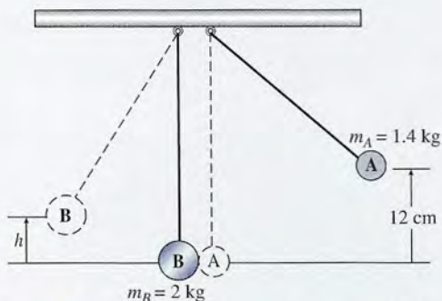
Figura 9.9 Colisión completamente elástica de dos bolas de metal suspendidas.
