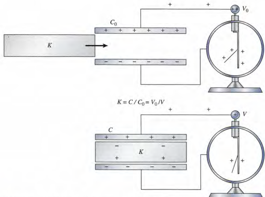
Figura 26.9 La inserción de un dieléctrico entre las placas de un condensador ocasiona una caída en la diferencia de potencial, lo que resulta en una mayor capacitancia.
