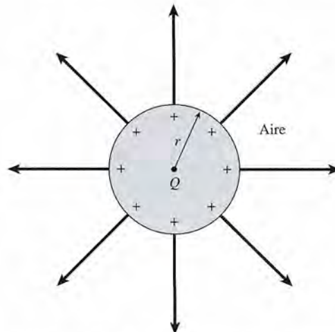
Figura 26.2 La cantidad de carga que puede transferirse a un conductor está limitada por la rigidez dieléctrica del medio circundante.
