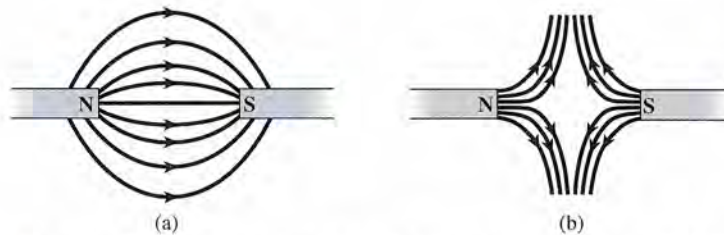
Figura 29.5 (a) Líneas de flujo magnético entre dos polos magnéticos diferentes. (b) Líneas de flujo magnético entre dos polos iguales.
