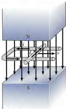
Figura 31.4 La fem inducida en un conductor de longitud L se mueve con una velocidad v perpendicular a un campo magnético \mathbf{B} .
