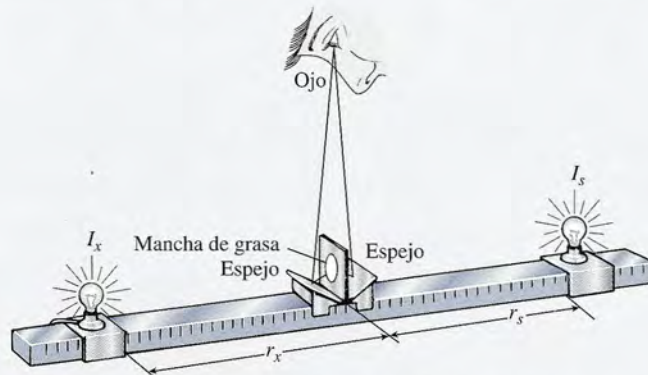
Figura 33.19 El fotómetro de mancha de aceite se usa para medir la intensidad de una fuente de luz desconocida, mediante la comparación con una fuente patrón (estándar).
