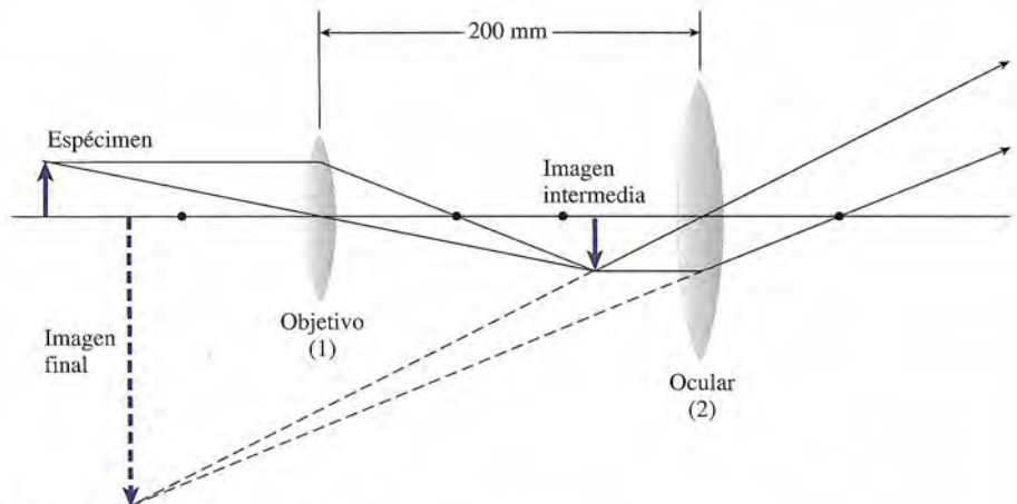
Figura 36.15 Combinaciones de lentes.
