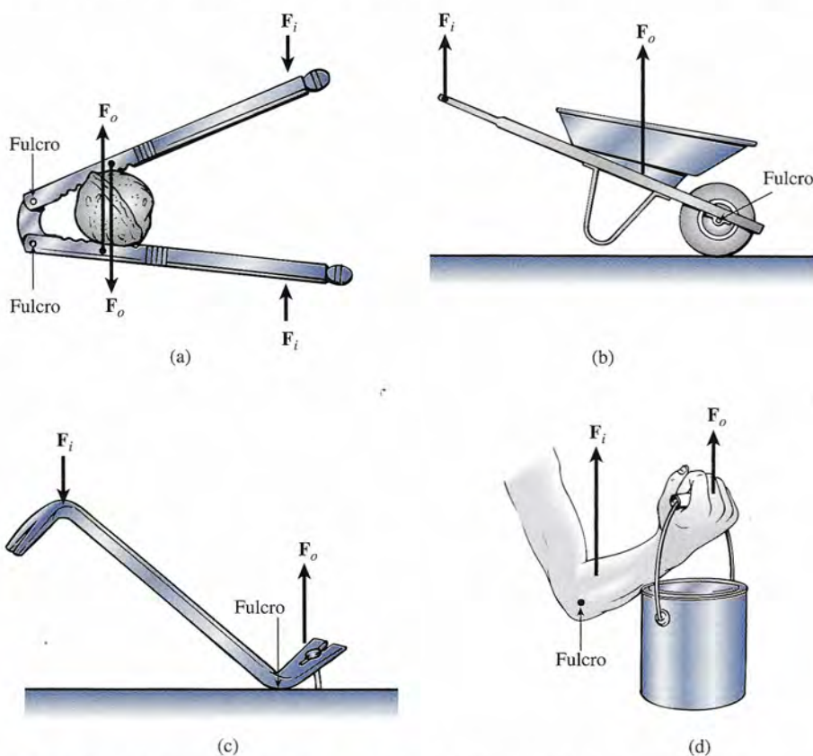
Figura 12.4 La palanca constituye el principio funcional de numerosas máquinas simples.
