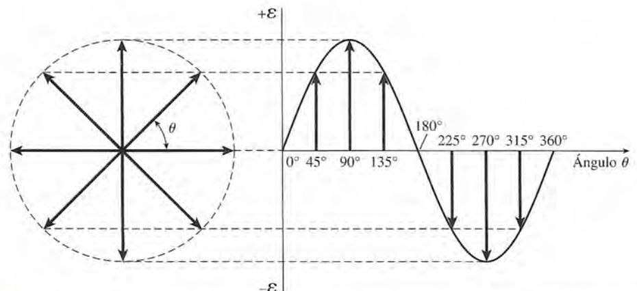
Figura 32.6 Es posible emplear un vector giratorio y su onda senoidal correspondiente para representar corriente o voltaje alternos (ca).
