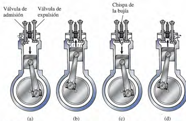
Figura 20.13 El motor de gasolina de cuatro tiempos: (a) carrera de admisión, (b) carrera de compresión, (c) carrera de trabajo y (d) carrera de expulsión.
