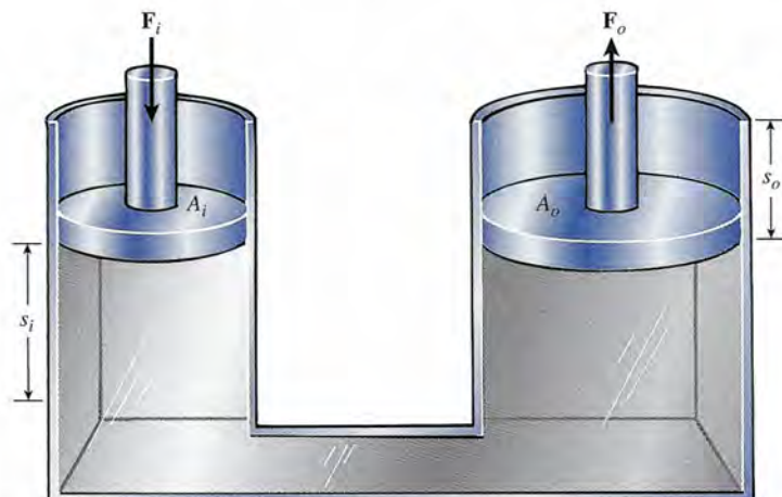
Figura 15.9 Prensa hidráulica.
