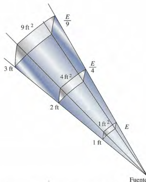
Figura 33.18 La intensidad luminosa I es constante para un ángulo sólido dado \Omega . Sin embargo, la iluminación E (flujo por unidad de área) disminuye en proporción al cuadrado de la distancia a la fuente de luz.
