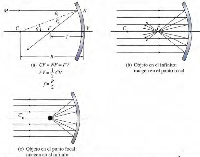
Figura 34.9 Punto focal de un espejo convergente (superficie cóncava): (a) la longitud focal es la mitad del radio de curvatura; (b) el objeto se encuentra en el infinito y la imagen en el punto focal; (c) el objeto está en el punto focal y la imagen en el infinito.
