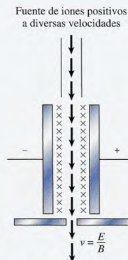
Figura 29.26 El selector de velocidad.
