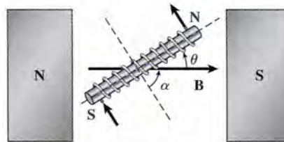
Figura 30.4 Momento de torsión magnético sobre un solenoide. El ángulo \alpha es el que forma cada espira de alambre con el campo \mathbf{B} . El ángulo \theta es el que se halla entre el eje del solenoide y ese mismo campo. Recuerde que \theta + \alpha = 90^\circ .
