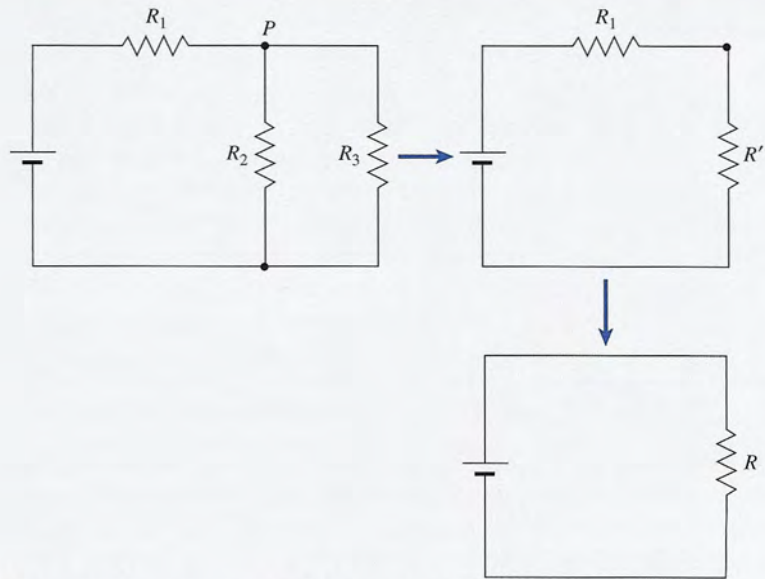
Figura 28.6 Reducción de un circuito complejo a un circuito equivalente simple.
