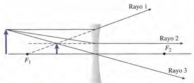
Figura 36.10 Principales rayos para construir la imagen formada por una lente divergente.
