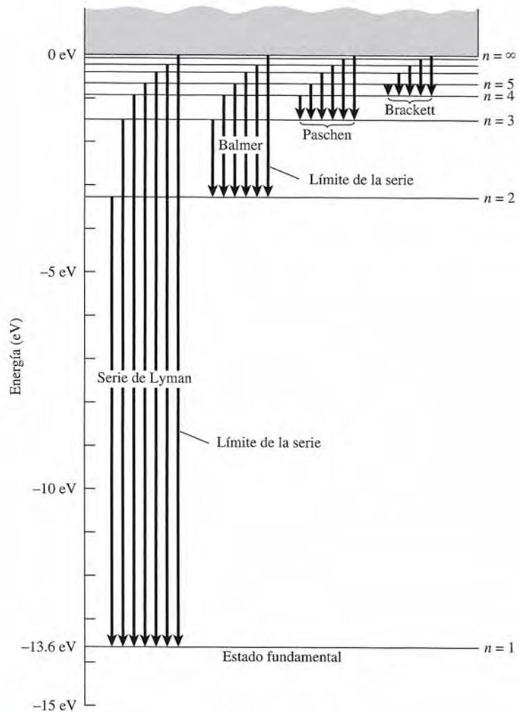
Figura 38.10 Diagrama de los niveles de energía del átomo de hidrógeno.
