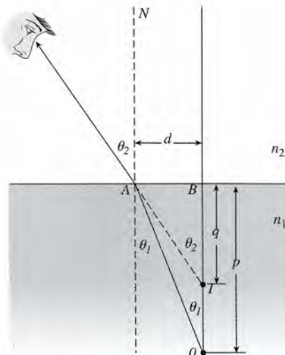
Figura 35.18 Relación entre la profundidad aparente y la profundidad real.
