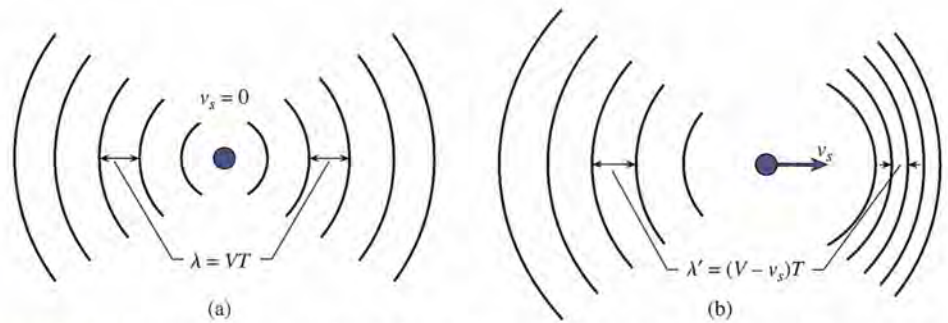
Figura 22.13 Cálculo de la magnitud de la longitud de onda del sonido emitido desde una fuente en movimiento. La velocidad de la fuente v_s se considera positiva para rapidez de acercamiento y negativa para rapidez de alejamiento.
