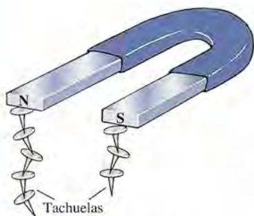
Figura 29.8 Inducción magnética.
