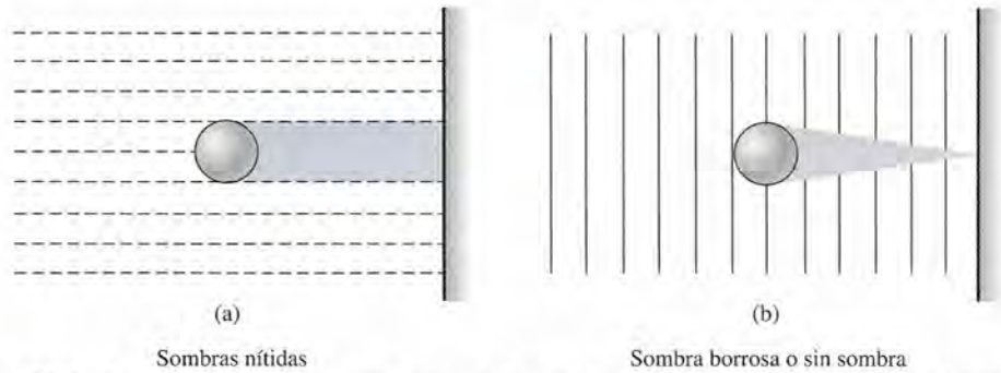
Figura 33.1 Un poderoso argumento en apoyo de la teoría corpuscular de la materia es la formación de sombras nítidas. Se sabe que las ondas se flexionan cuando encuentran obstáculos en su trayectoria.
