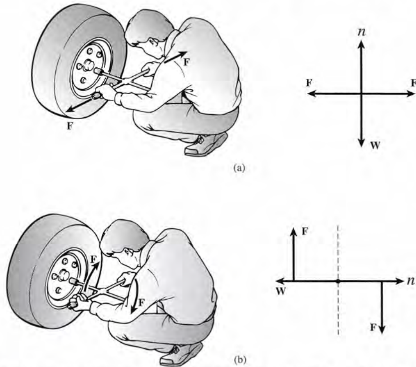
Figura 5.1 (a) Hay equilibrio puesto que las fuerzas tienen la misma línea de acción. (b) No hay equilibrio porque las fuerzas opuestas no tienen la misma línea de acción.
