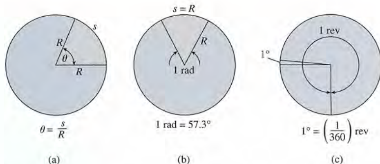
Figura 11.2 Medida del desplazamiento angular y una comparación de unidades.
