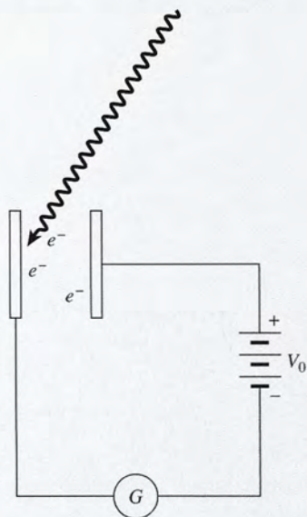
Figura 38.14 El potencial de frenado V_0 es la diferencia de potencial que retarda la transición de los fotoelectrones con más energía, proyectados a causa de la radiación incidente.
