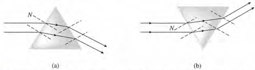
Figura 36.1 Los rayos paralelos de luz se flexionan hacia la base del prisma y permanecen paralelos.
