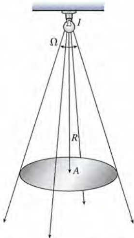
Figura 33.16 Cálculo de la iluminación de una superficie perpendicular al flujo luminoso incidente.
