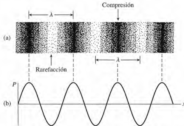
Figura 22.3 (a) Compresiones y rarefacciones de una onda de sonido en el aire en un instante específico. (b) La variación senoidal de la presión en función del desplazamiento.
