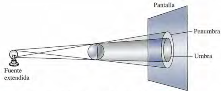
Figura 33.12 Sombras formadas por una fuente de luz extendida.
