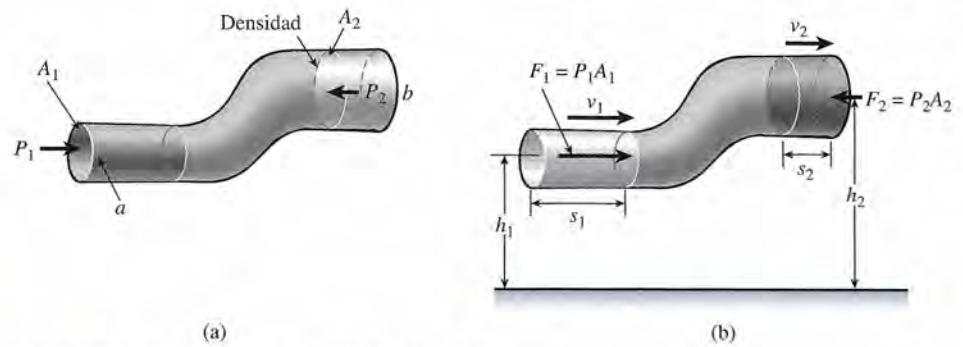
Figura 15.17 Deducción de la ecuación de Bernoulli.
