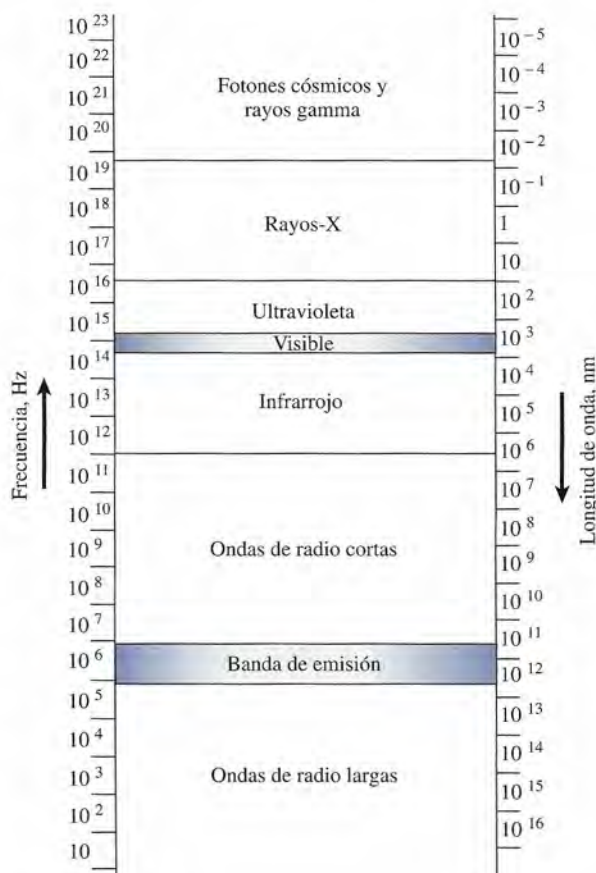
Figura 33.7 Espectro electromagnético.
