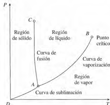
Figura 19.8 Diagrama de fases del punto triple para el agua o cualquier otra sustancia que se dilate al congelarse.
