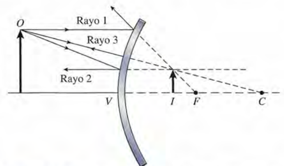
Figura 34.12 Principales rayos para la construcción gráfica de las imágenes reflejadas por espejos divergentes (convexos).
