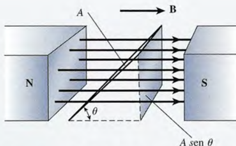
Figura 29.10 Cálculo del flujo magnético a través de una espira rectangular.
