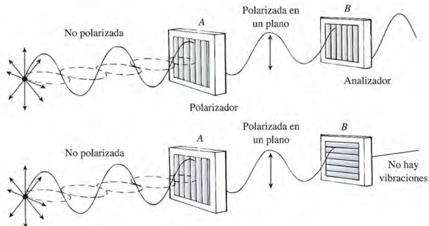
Figura 37.15 Analogía mecánica para explicar la polarización de una onda transversal.
