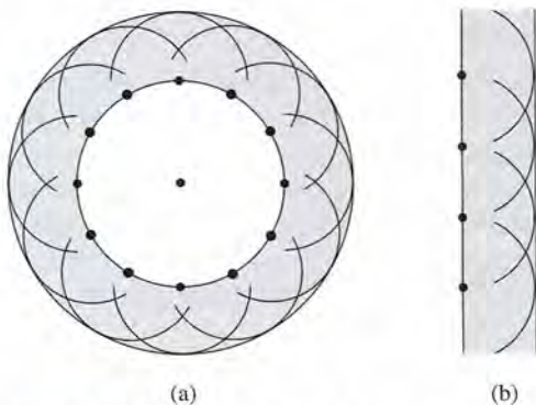
Figura 33.2 El principio de Huygens (a) para una onda esférica y (b) para una onda plana.
