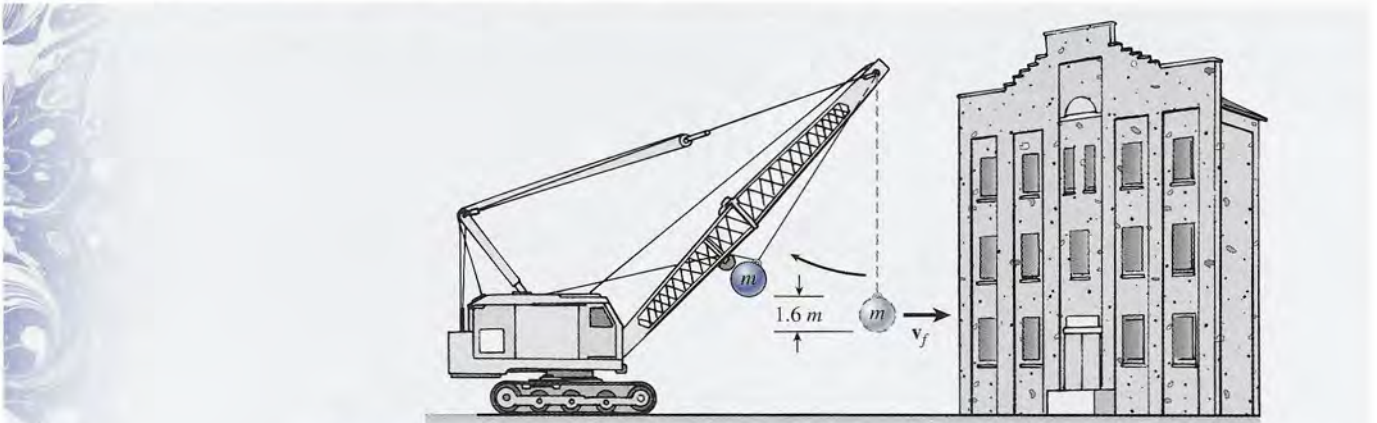
Figura 8.8 La velocidad de una masa suspendida al pasar por el punto más bajo de su trayectoria puede determinarse a partir de las consideraciones generales sobre la energía.
