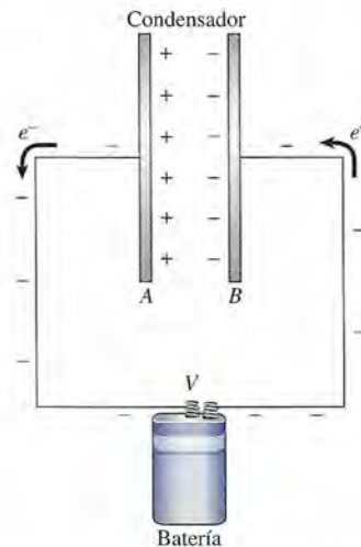
Figura 26.5 Carga de un condensador mediante la transferencia de carga de una placa a otra.
