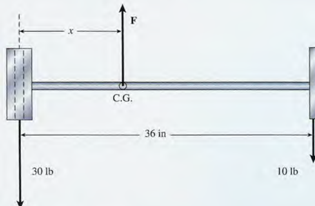
Figura 5.10 Cálculo del centro de gravedad.
