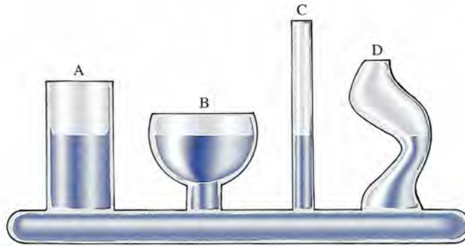
Figura 15.5 El agua siempre busca su propio nivel, lo cual indica que la presión es independiente del área o de la forma del recipiente.
