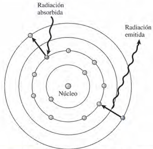
Figura 33.9 El histórico átomo de Bohr es una manera útil de visualizar las transiciones entre los niveles de energía.
