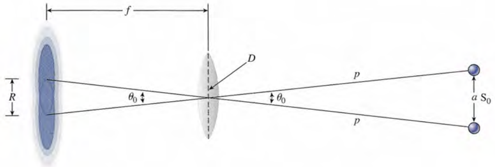
Figura 37.14 Resolución de dos objetos distantes por medio de una lente esférica.
