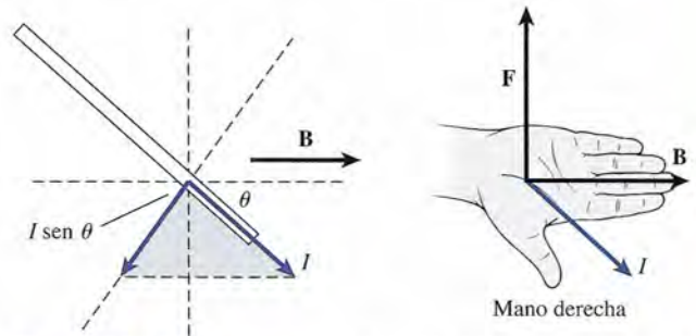
Figura 29.19 La fuerza magnética sobre un conductor por el cual circula una corriente. La corriente está dirigida a un ángulo \theta respecto al campo \mathbf{B} .
