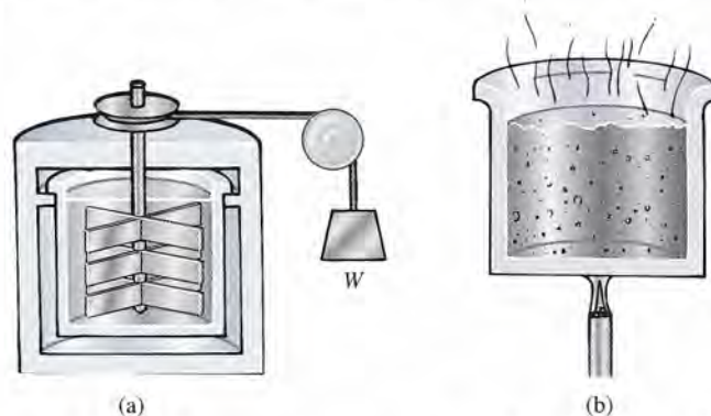
Figura 20.1 Aumento de la energía interna de un sistema (a) realizando trabajo y (b) suministrando calor al sistema.
