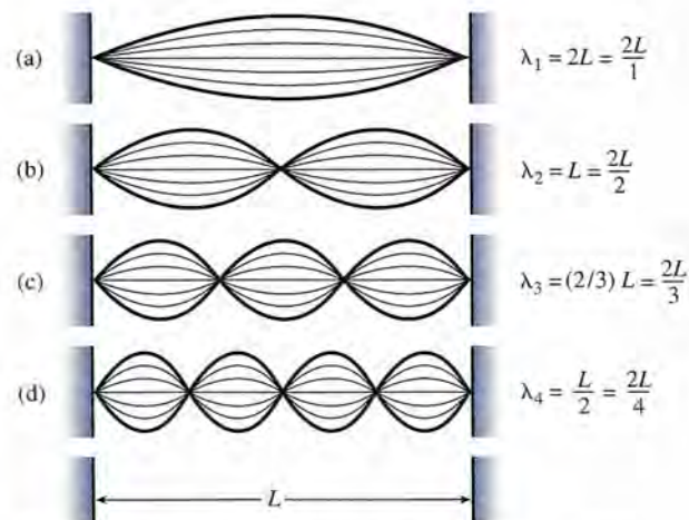
Figura 21.12 Modelos posibles de ondas estacionarias en una cuerda vibrante.
