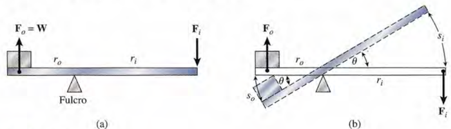
Figura 12.3 La palanca.
