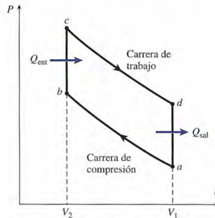
Figura 20.14 El ciclo de Otto de un motor de gasolina de cuatro tiempos.
