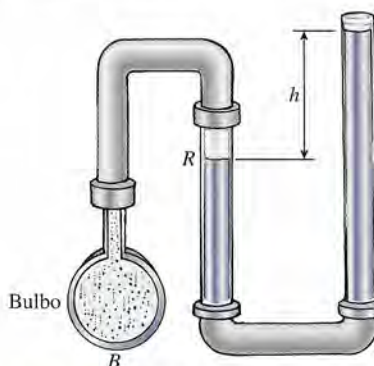
Figura 16.6 Termómetro a volumen constante.
