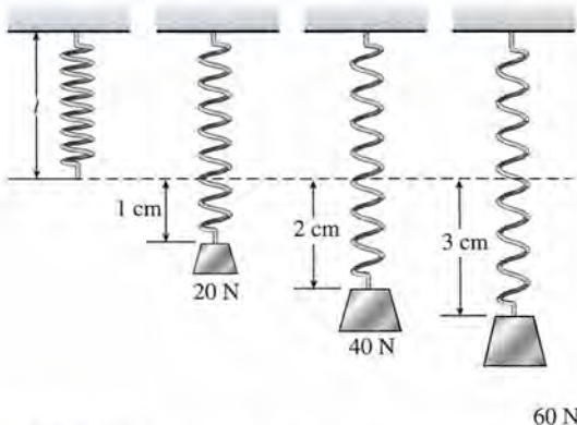
Figura 13.1 Alargamiento uniforme de un resorte.
