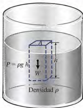
Figura 15.4 Relación entre presión, densidad y profundidad.
