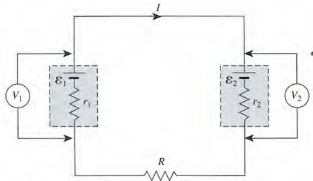
Figura 28.8 Inversión de la corriente mediante una fuente de fem.
