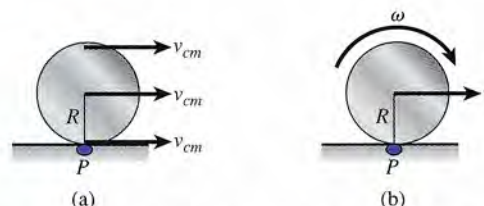
Figura 11.10 (a) Todas las partes de un disco en traslación pura se mueven con la velocidad v_{cm} del centro de masa. (b) Un objeto rodando es una combinación de traslación y rotación de tal forma que la velocidad lineal horizontal está dada por v = \omega R .
