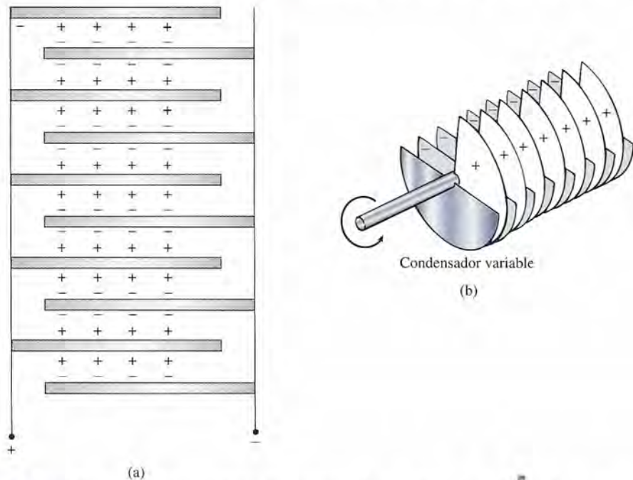
Figura 26.7 (a) Un condensador está formado de varias placas apiladas que alternan las cargas positiva y negativa. (b) En un condensador variable uno de los juegos de placas gira con relación a otro, lo que ocasiona un cambio en el área real.
