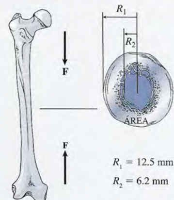
Figura 13.9 Esfuerzo de compresión en el hueso del muslo (fémur). (Figura por Hemera, Inc.)
