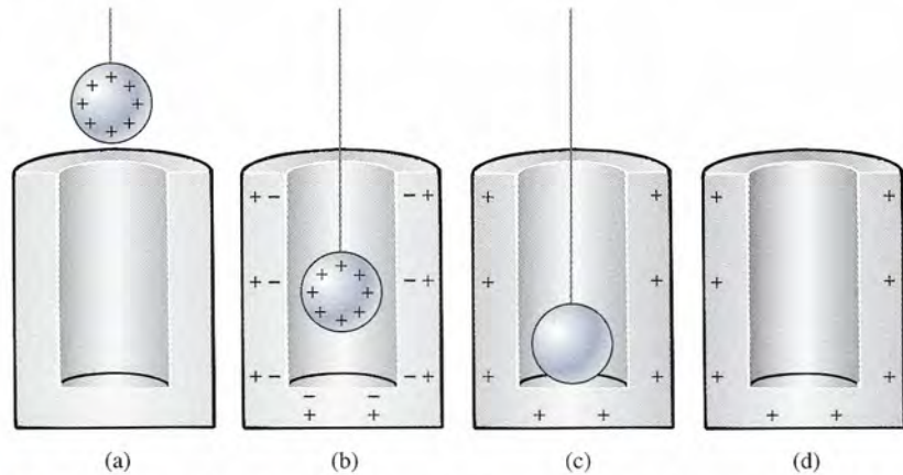
Figura 24.13 El experimento de Faraday demuestra la redistribución de la carga neta sobre las paredes del conductor metálico hueco.
