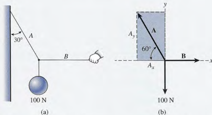
Figura 4.9 Las fuerzas que actúan en el nudo se representan en un diagrama de cuerpo libre.
