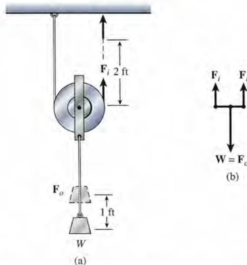
Figura 12.7 Una polea simple móvil. (a) La fuerza de entrada se mueve a lo largo de una distancia igual al doble de la distancia que recorre la fuerza de salida. (b) El diagrama de cuerpo libre muestra que 2F_i = F_o .
