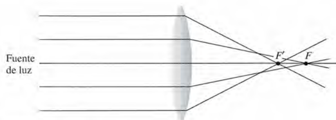
Figura 36.17 Aberración esférica.
