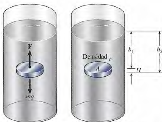
Figura 15.10 El empuje que se ejerce sobre el disco es igual al peso del fluido que se desplaza.
