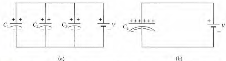
Figura 26.12 Capacitancia equivalente de un conjunto de condensadores conectados en paralelo.
