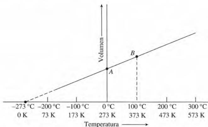
Figura 19.3 Variación del volumen como función de la temperatura. Cuando el volumen se extrapola a cero, la temperatura de un gas es la del cero absoluto (0 K).
