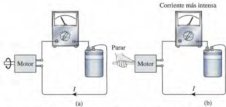
Figura 31.13 Demostración de la existencia de una fuerza contraelectromotriz en un motor de cd. Parar el motor reduce la fuerza contraelectromotriz a cero y esto aumenta la corriente del circuito.
