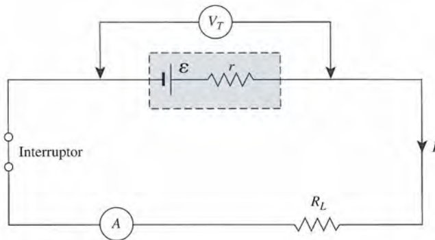
Figura 28.7 Resistencia interna.
