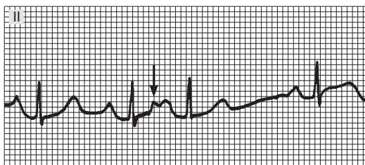
Extrasístole auricular
