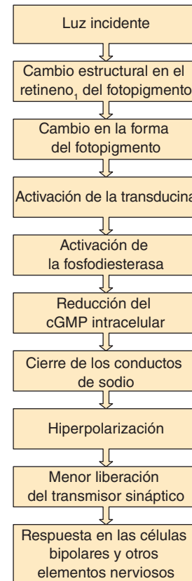
FIGURA 12-15 Secuencia de acontecimientos que participan en la fototransducción de los bastones y los conos. cGMP, monofosfato de guanosa cíclico.
