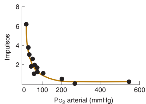
FIGURA 37-6 Efecto de la P_{CO_2} en las descargas del nervio aferente. Se grafica la velocidad de descarga de una sola fibra aferente del cuerpo carotídeo con varias P_{O_2} (círculos) y se adapta a una línea. Se observa aumento marcado en la velocidad de descarga conforme P_{O_2} cae por debajo de los niveles de reposo normales (o sea, cerca de 100 mmHg). (Por cortesía de S. Sampson.)
