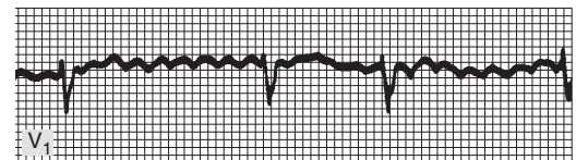
Fibrilación auricular
