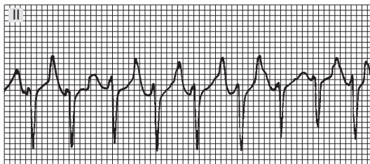
Taquicardia auricular
