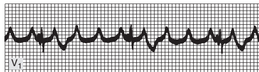
Flúter auricular
