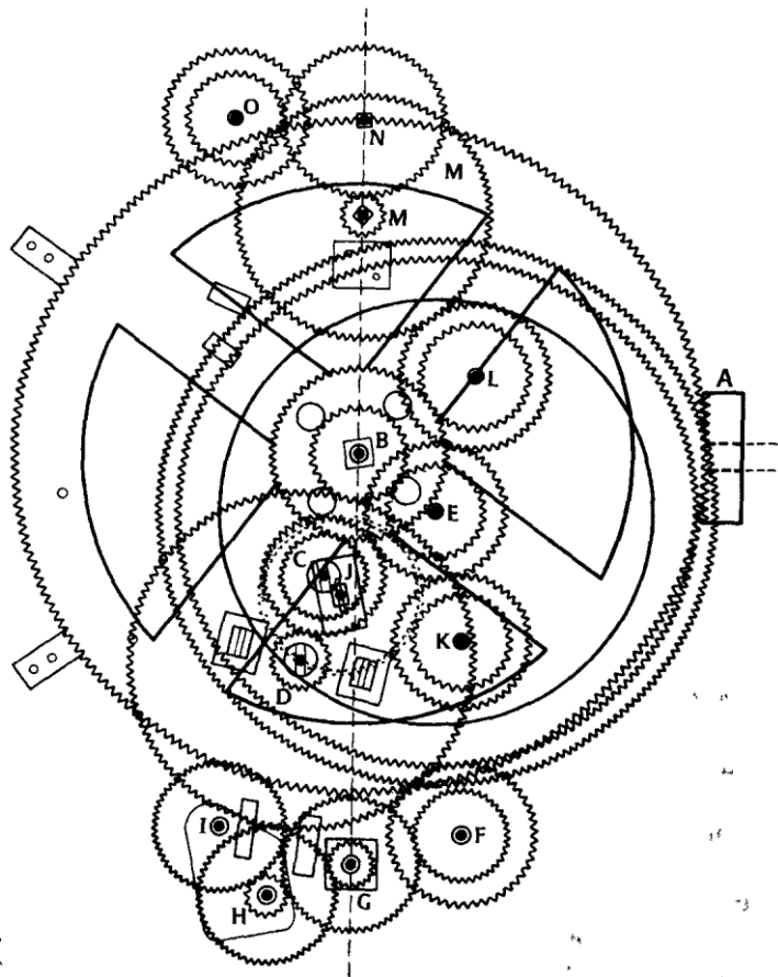
El engranaje de Anticitera (Según el dibujo de B. Pope en Price, Gears , p. 37, fte. 29, reproducida con autorización de la American Philosophical Society .)
