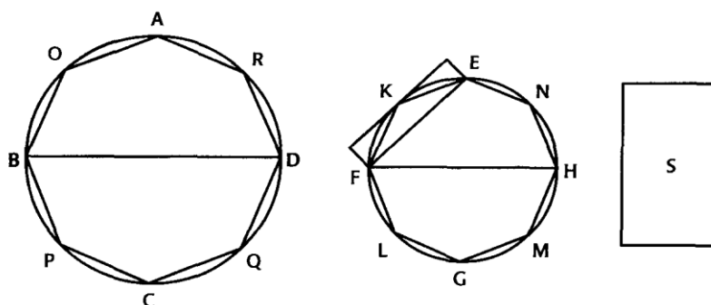
Demostración de Euclides por el método de la exhaustión. (Basada en Thomas, Greek Mathematical Works , i. 461)
